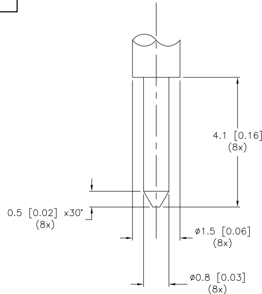
DETAIL A SCALE: 1=4
